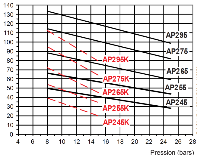
Débit (l/h) Débit de la pompe
